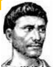
250 AD Diophantus
